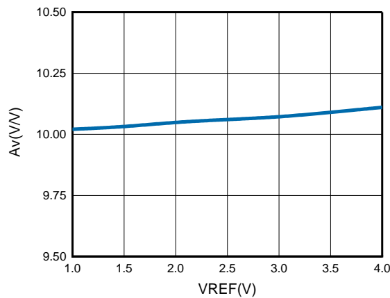
Figure 5. AV vs. VREF
