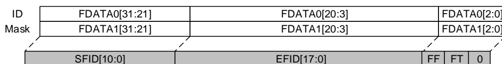
图 26-7. 32-bit 位宽掩码模式过滤器
