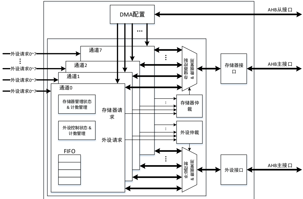
图 10-1. 系统架构
