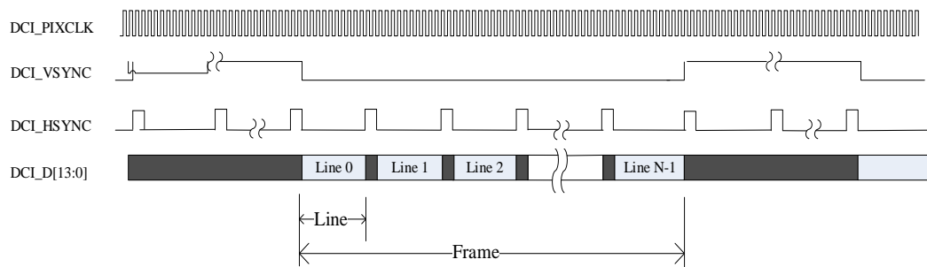
图 22-2. 硬件同步模式
