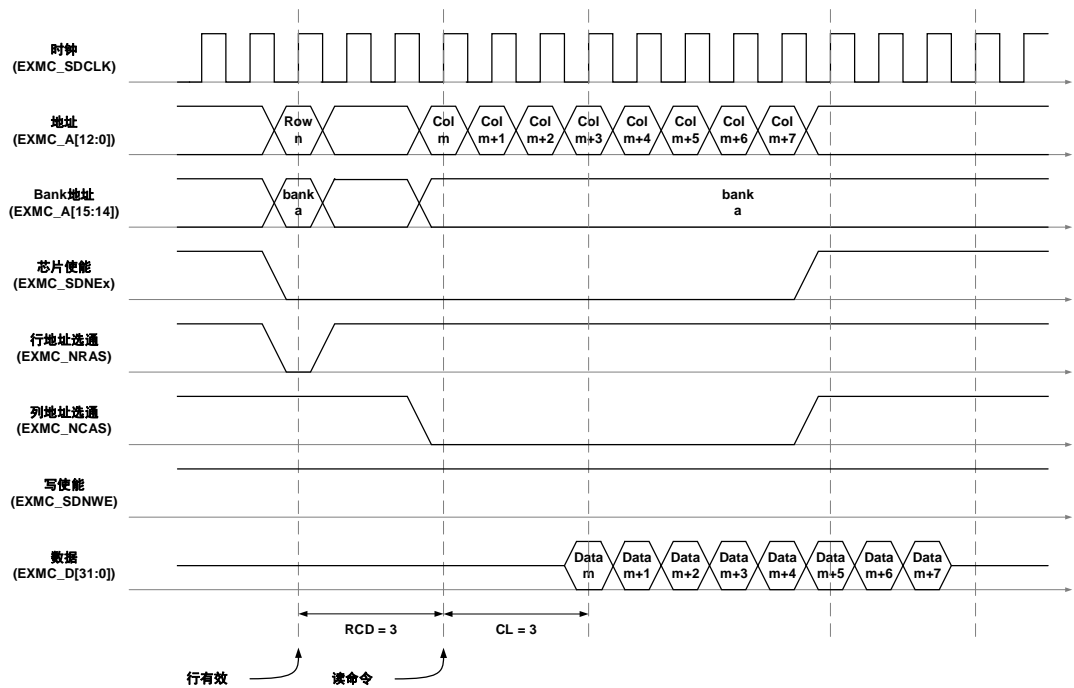
图 25-30. 突发读操作
