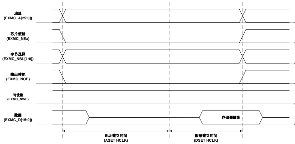
图 25-8. 模式 1 写时序
