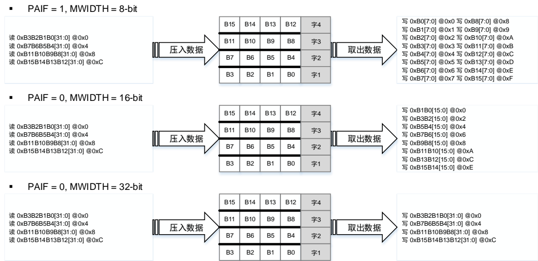
图 10-6. PWIDTH 为‘2b10’时，数据的打包/解包
