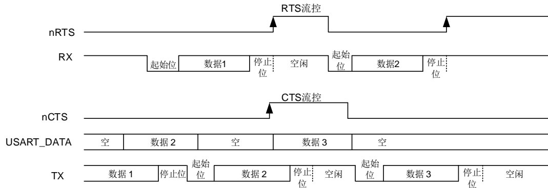
图 19-8. 硬件流控制
