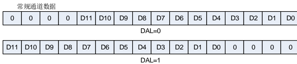
图 14-8. 10 位数据存储模式
