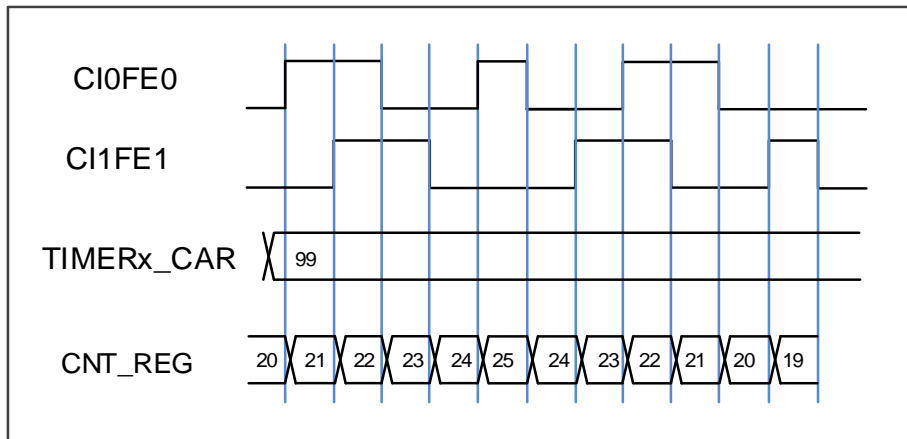
图 18-19. 在译码器模式 2 且 CI0FE0 极性反相时计数器行为
