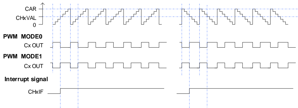
图 18-38. EAPWM 时序图
