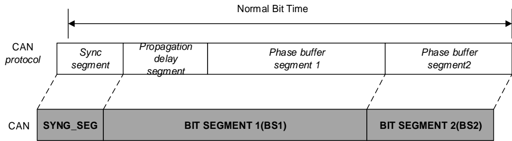
图 26-11. 位时序
