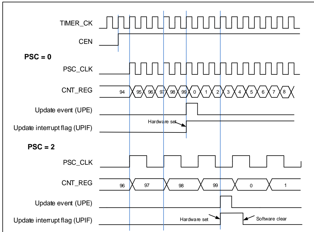
图 18-59. 向上计数时序图, PSC=0/2
