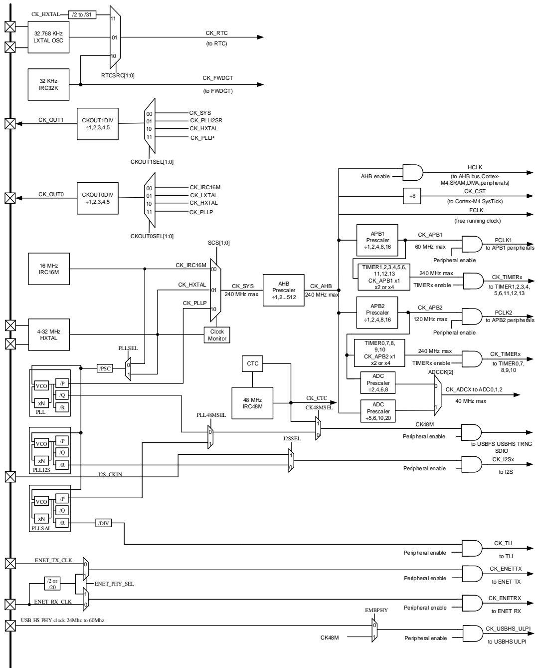
图 4-2. 时钟树
