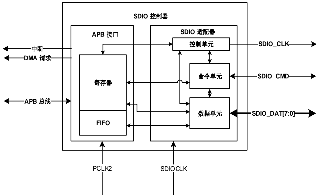
图 24-6. SDIO 框图
