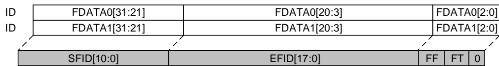
图 26-9. 32-bit 位宽列表模式过滤器
