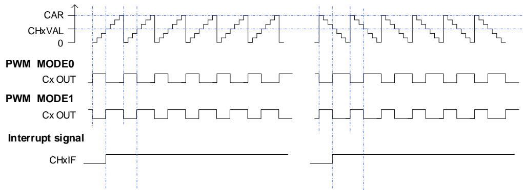
图 18-51. CAPWM 时序图
