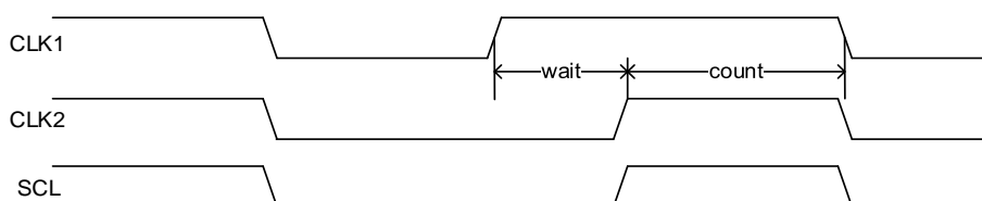
图 20-4. 时钟同步
