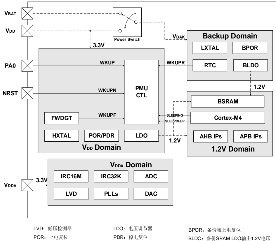
图 3-1. 电源域概览
