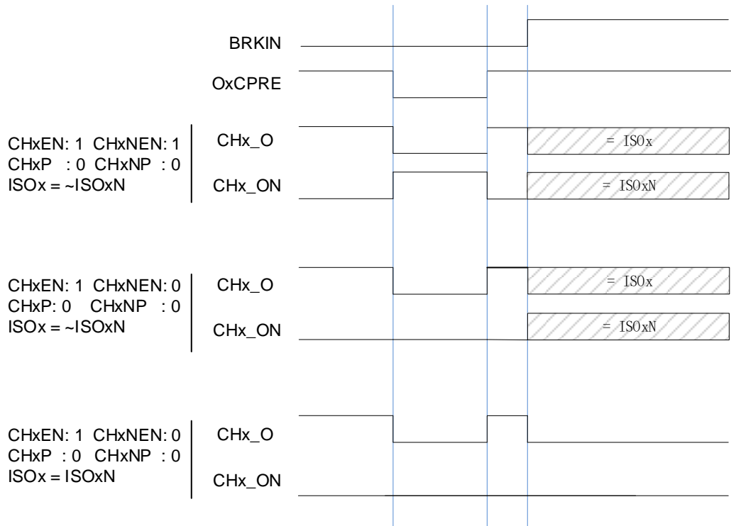
图 18-17. 通道响应中止输入（高电平有效）时，输出信号的行为
