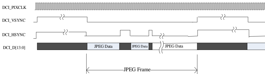
图 22-3. 硬件同步模式之 JPEG 格式
