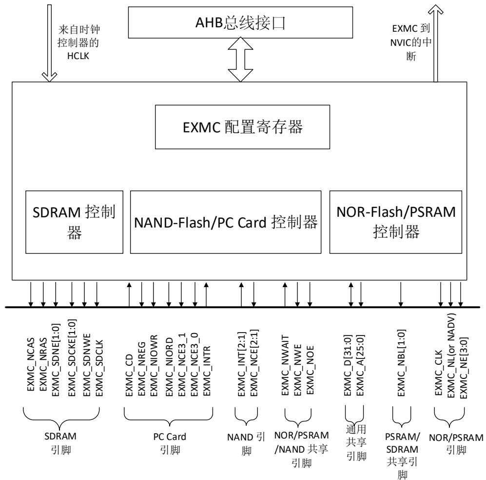
图 25-1. 系统架构
