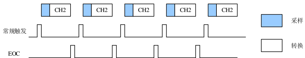
图 14-2. 单次运行模式
