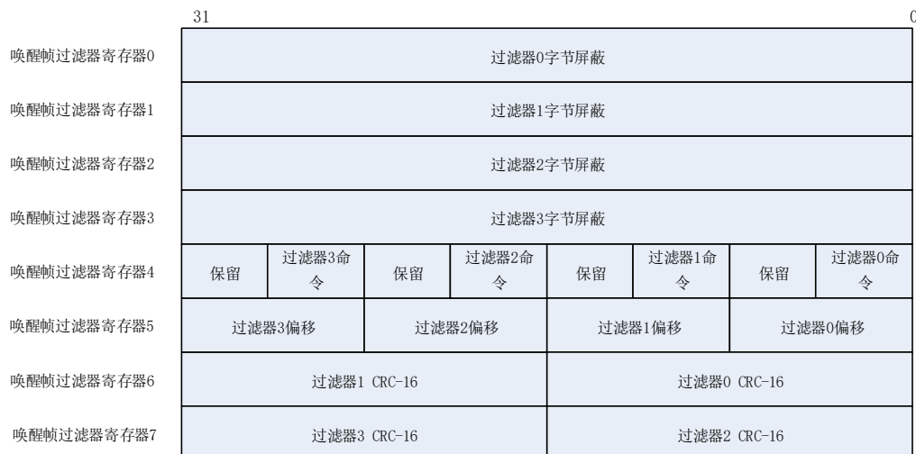
图 27-15. 远程唤醒帧过滤器寄存器
