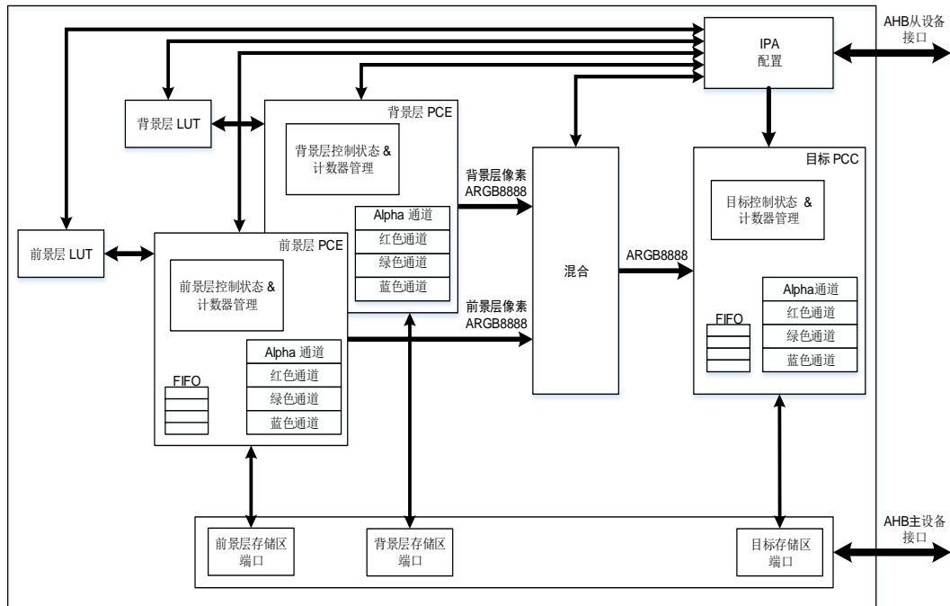
图 11-1. IPA 模块框图
