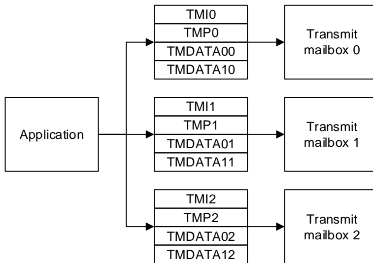
图 26-2. 发送寄存器
