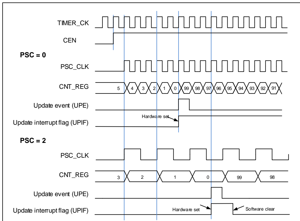
图 18-33. 向下计数时序图，PSC=0/2
