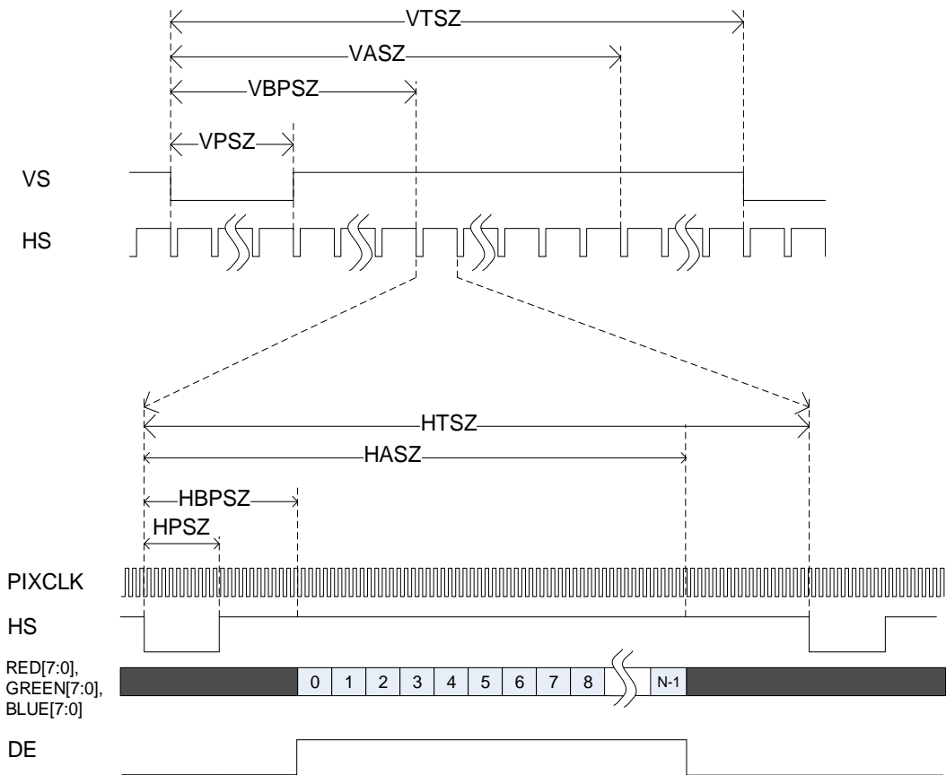
图 23-2. 显示时序图
