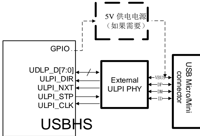
图 29-4. 使用外部 ULPI PHY 的连接示意图
