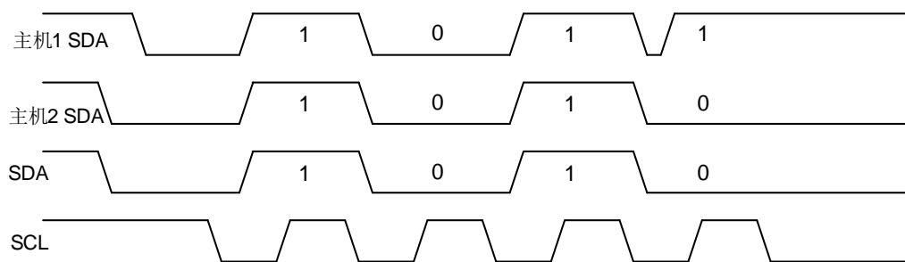
图 20-5. SDA 线仲裁
