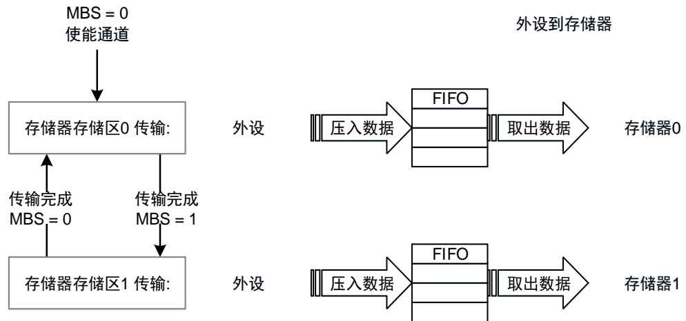
图 10-7. 存储切换模式
