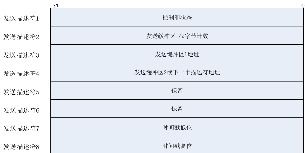
图 32-8. 增强发送描述符
