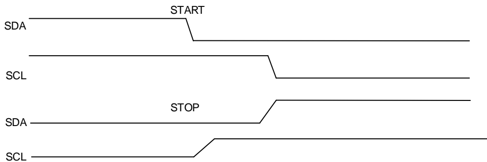
图 24-16. 开始和停止信号
