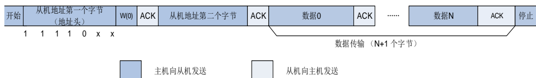
图 24-17. 10 位地址的 I2C 通讯流程（主机发送）
