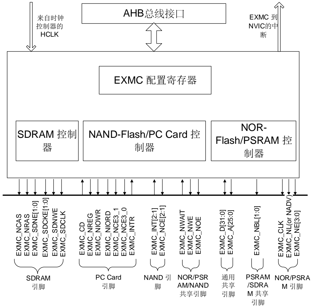
图 30-1. 系统架构
