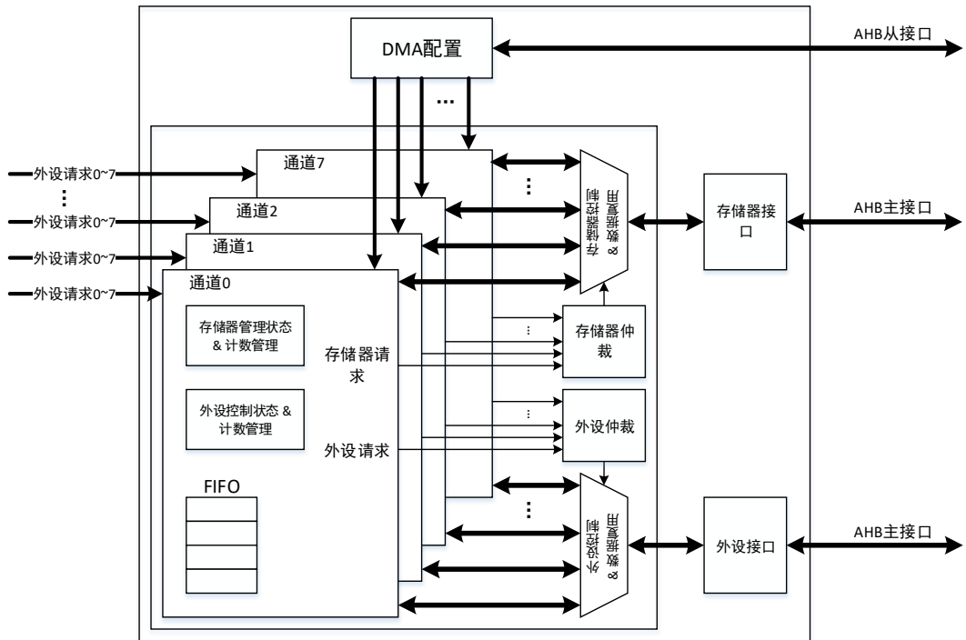
图 14-1. 系统架构
