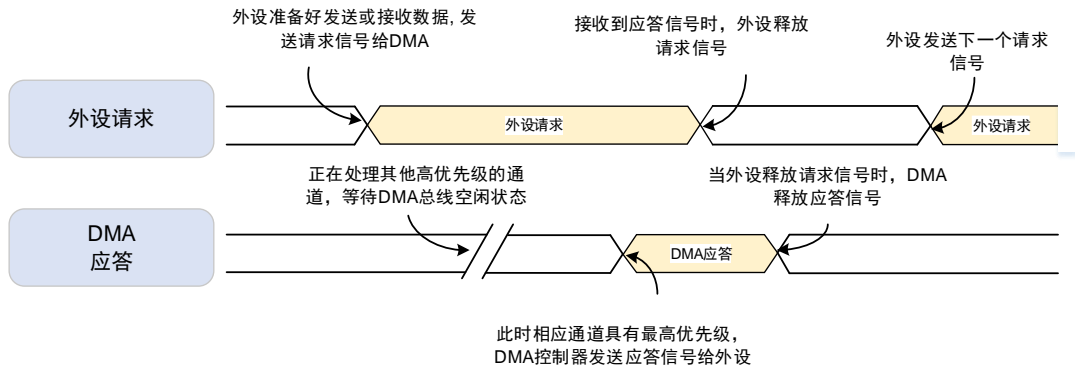
图 14-3. 握手机制
