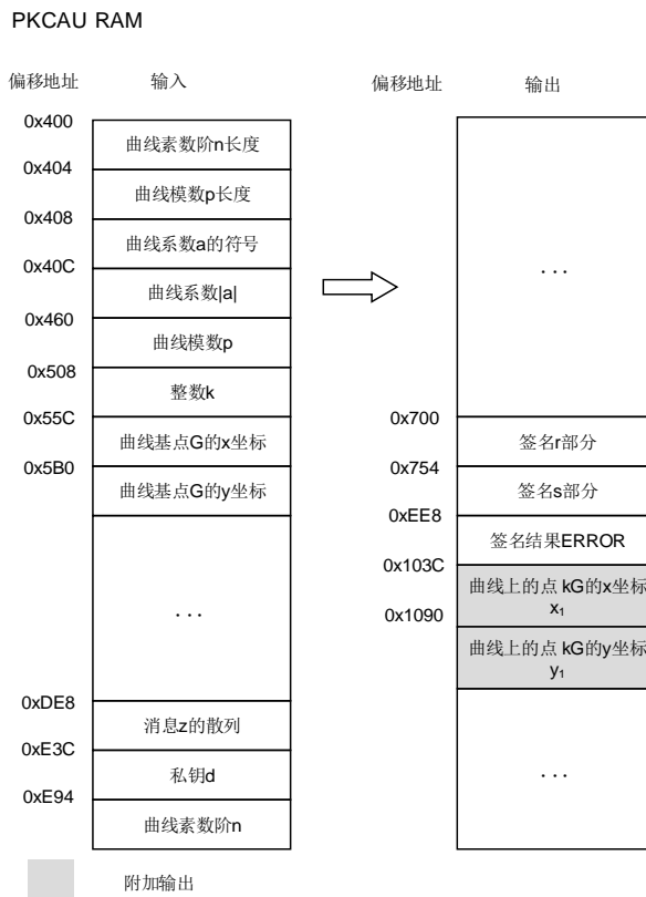
图 11-22. ECDSA 签名
