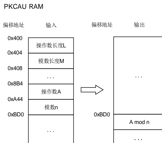
图 11-9. 取模运算
