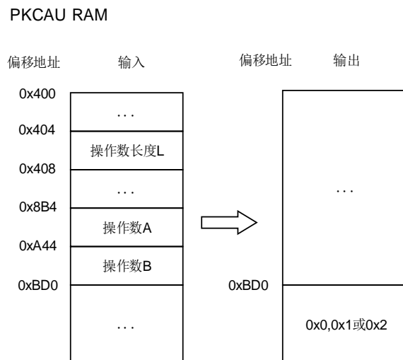
图 11-8. 算术比较
