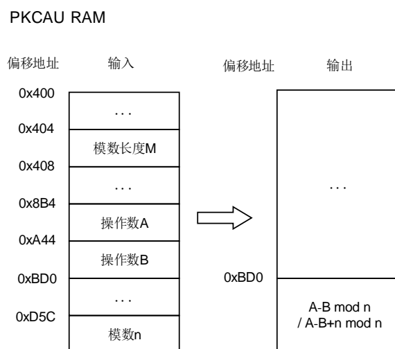
图 11-11. 模减法
