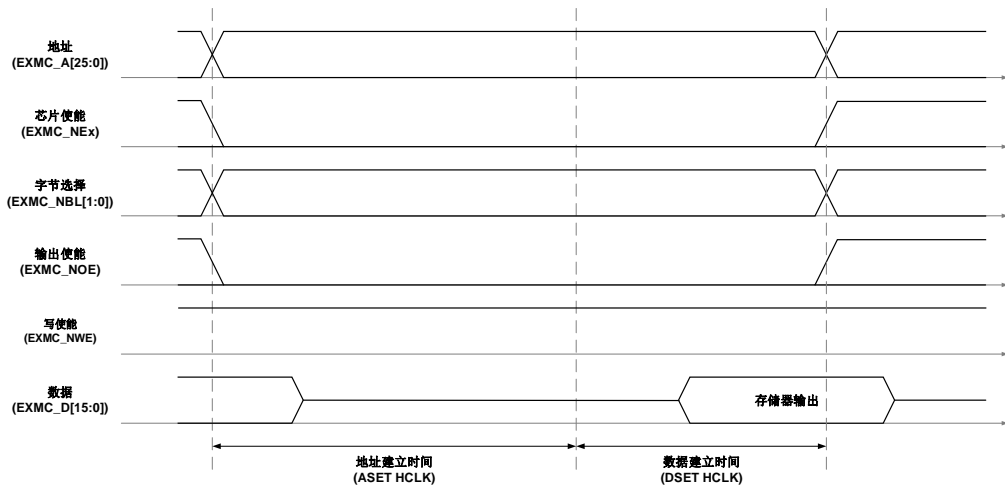
图 30-8. 模式 1 写时序
