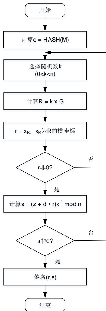
图 11-3. ECDSA 签名流程图
