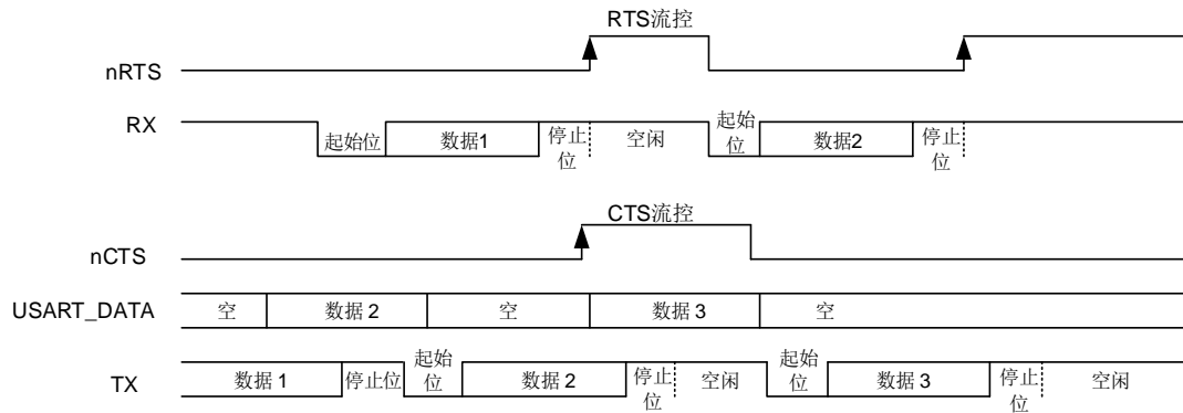
图 23-8. 硬件流控制
