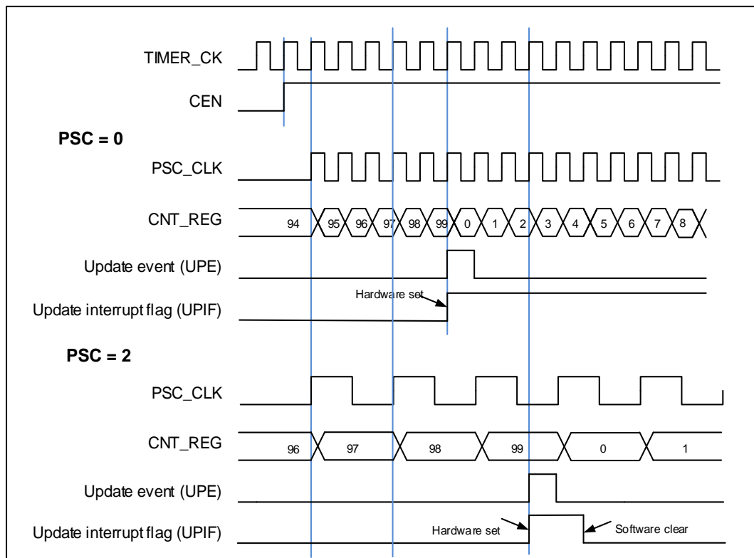
图 22-72. 向上计数时序图，PSC=0/2
