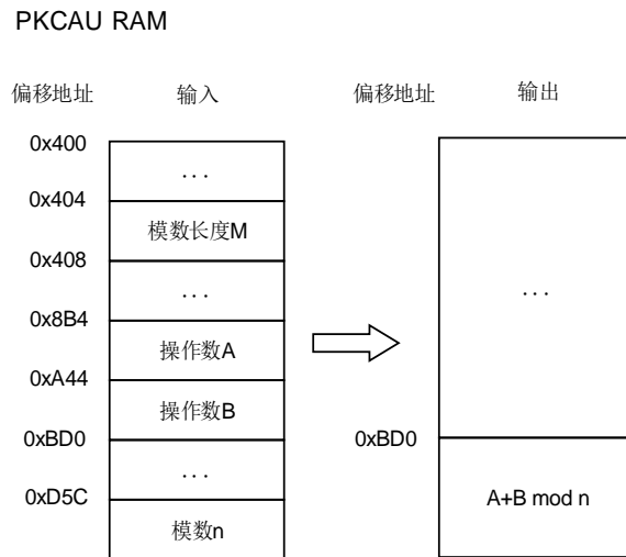
图 11-10. 模加法
