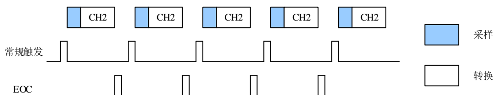
图 18-2. 单次运行模式
