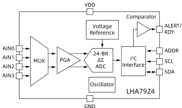
简化框图
