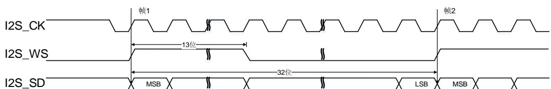
图 21-46. PCM 标准长帧同步模式时序图 (DTLEN=10, CHLEN=1, CKPL=1)
