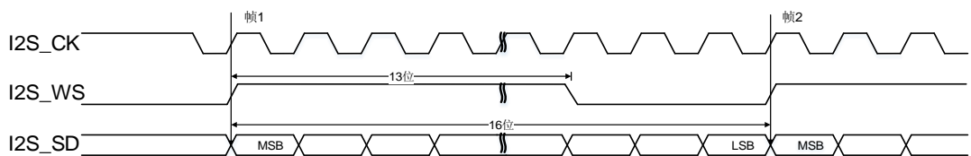
图 21-44. PCM 标准长帧同步模式时序图 (DTLEN=00, CHLEN=0, CKPL=1)
