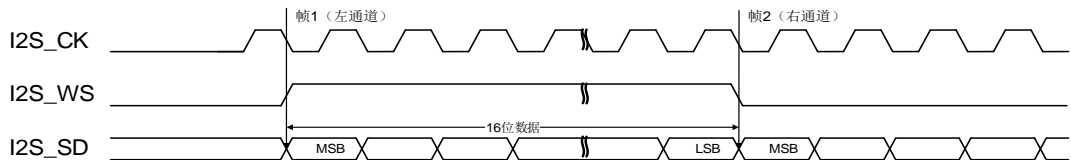
图 21-24. MSB 对齐标准时序图 (DTLEN=00, CHLEN=0, CKPL=1)
