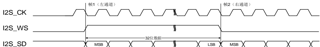
图 21-25. MSB 对齐标准时序图 (DTLEN=10, CHLEN=1, CKPL=0)
