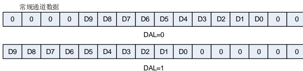
图 14-8. 10 位数据存储模式
