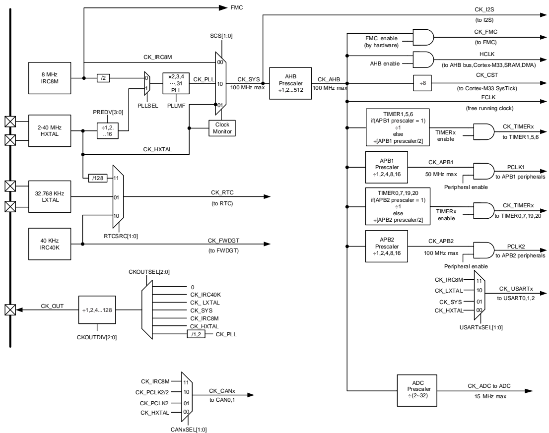
图5-2. 时钟树
