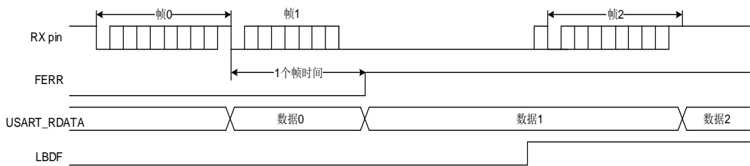
图 19-10. 数据传输过程中检测断开帧
