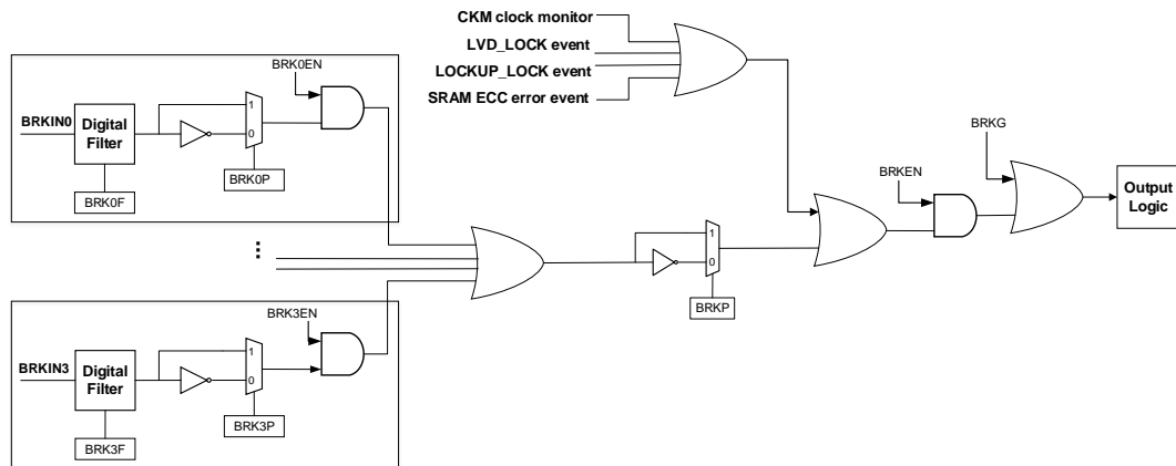
图 18-29 中止功能图
