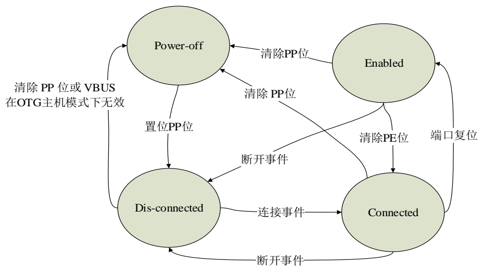
图 29-5. 主机端口状态转移图
