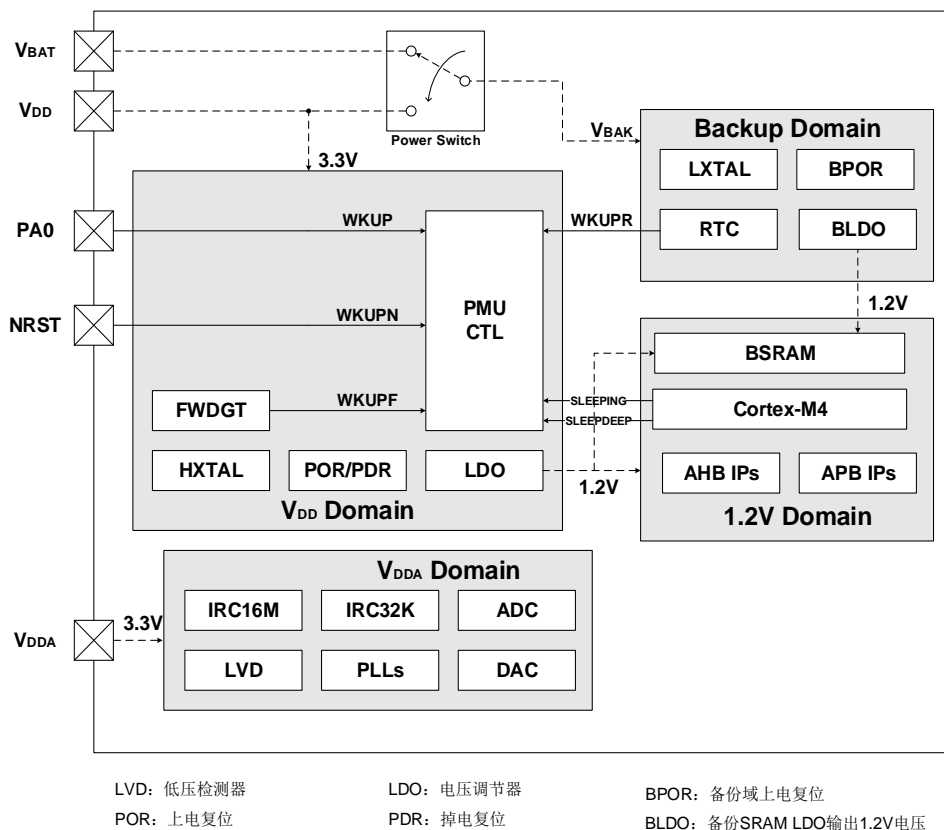
图3-1. 电源域概览
