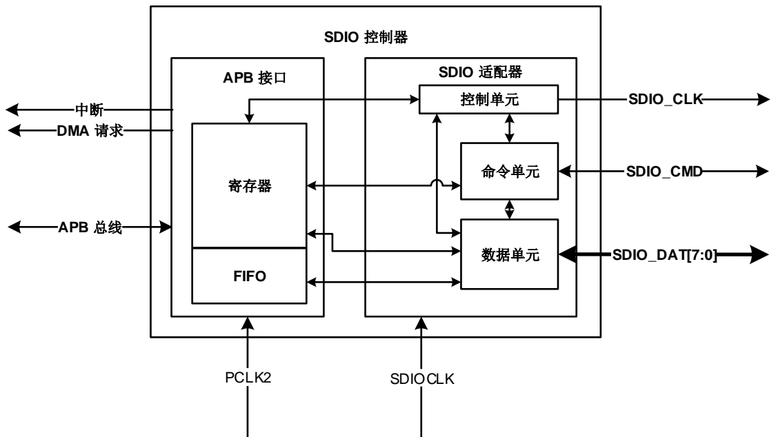
图 24-6. SDIO 框图
