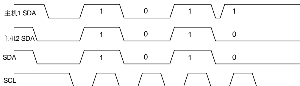
图 20-5. SDA 线仲裁
