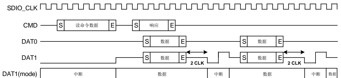
图 24-17. 4 位模式下多块读中断周期时序
