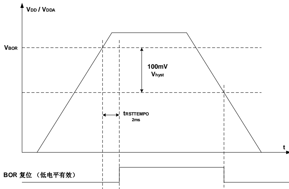
图3-3. BOR波形图
