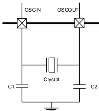
图4-3. HXTAL时钟源
