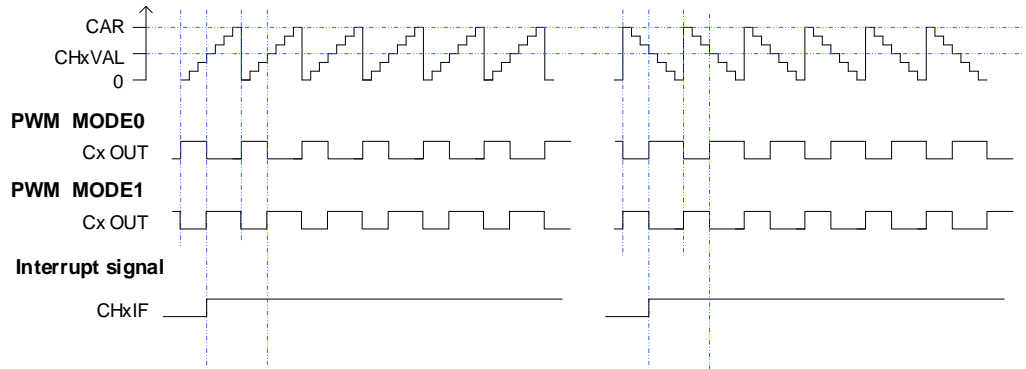
图 18-51. CAPWM 时序图
